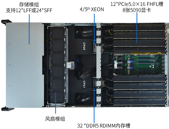
内部构造图
