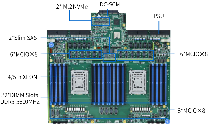
主板
