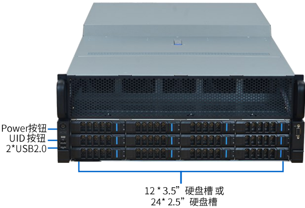
正视图
