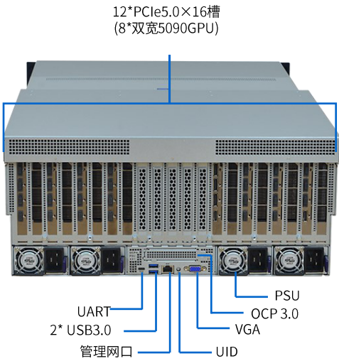
后视图
