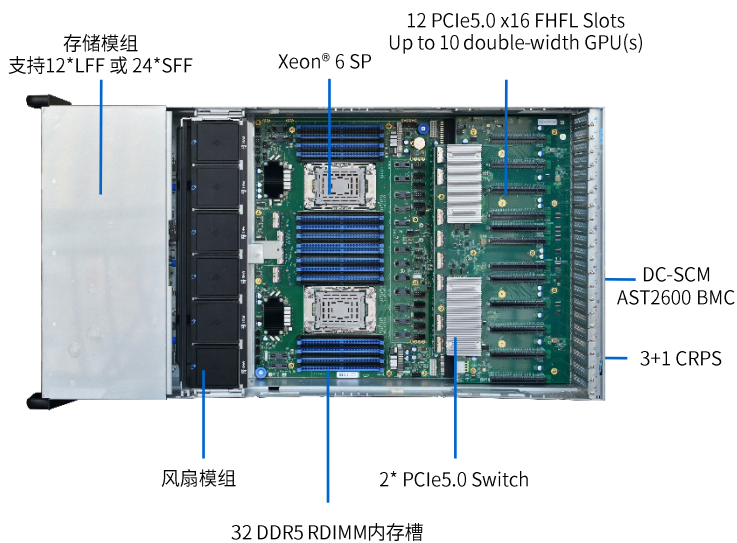
内部构造图
