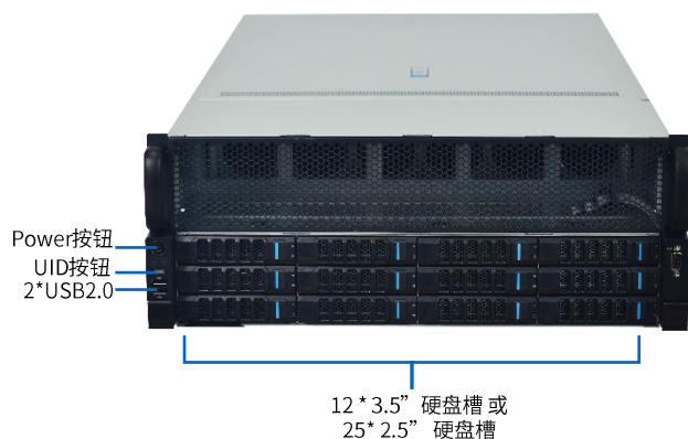
正视图
