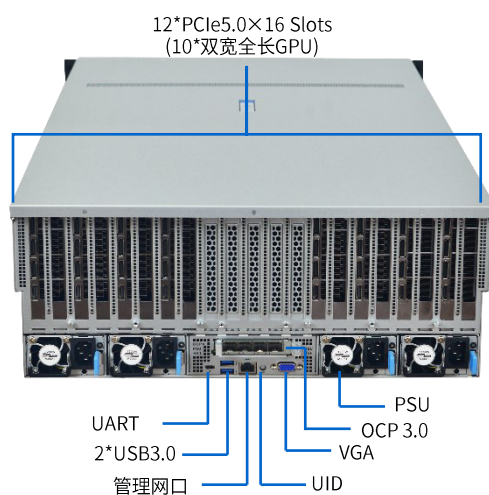
后视图
