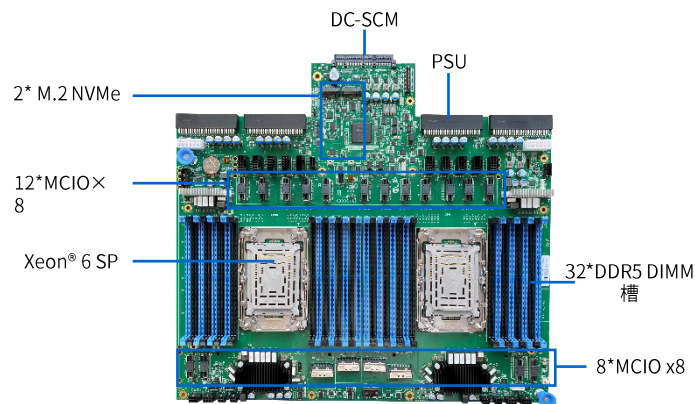
主板
